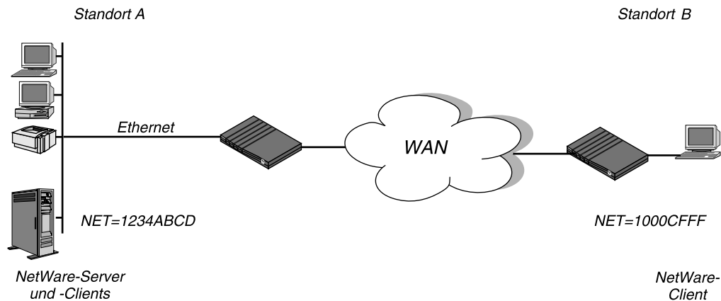
Abbildung 8-3: Einwahl-Client, der in sein eigenes IPX-Netzwerk eingebunden ist
