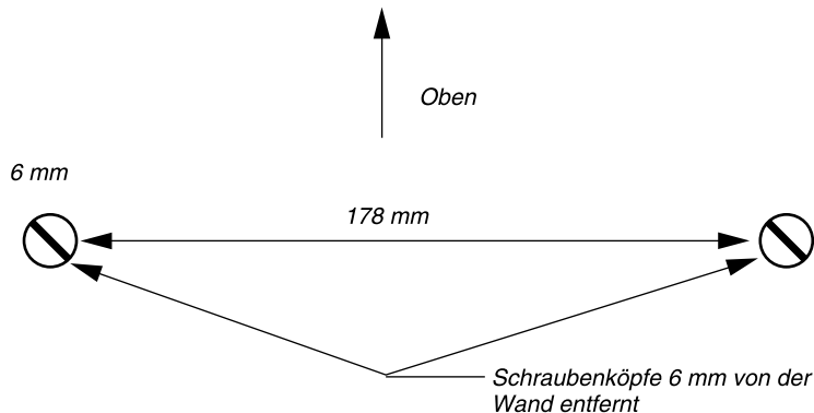
Abbildung 2-18: Position der Schrauben für die Wandmontage der Pipeline
