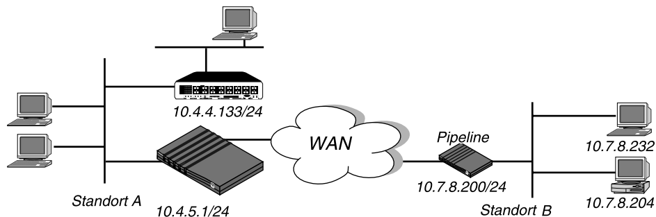
Abbildung 7-10: Verbindung zwischen lokalen und entfernten Subnetzen
