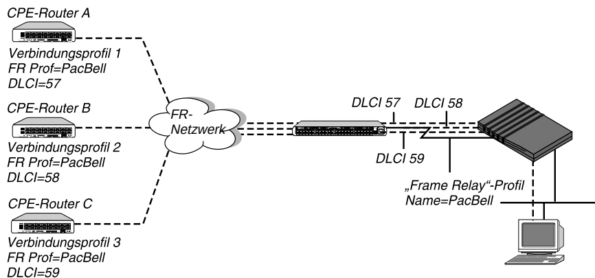
Abbildung 5-2: Gateway-Verbindungen zum Frame-Relay-Netzwerk
