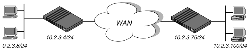
Abbildung 6-5: Beispiel für eine IP Bridging-Verbindung
