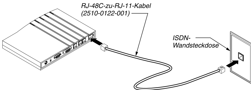
Abbildung 2-3: Verbinden einer Pipeline mit U-Schnittstelle mit dem ISDN-Anschluß
