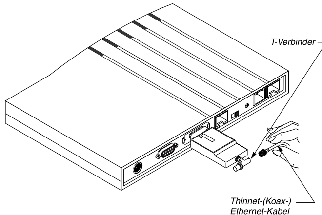
Abbildung 2-9: Anschließen des Thinnet-Kabels
