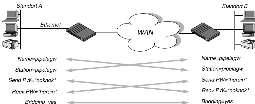
Abbildung 6-1: Aushandeln einer Bridging-Verbindung (PPP-Einkapselung)
