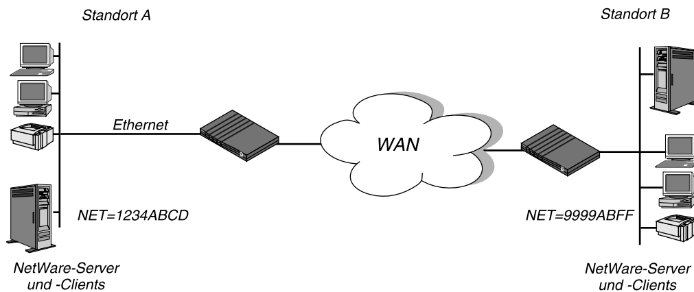
Abbildung 8-2: Verbindung mit NetWare-Servern auf beiden Seiten
