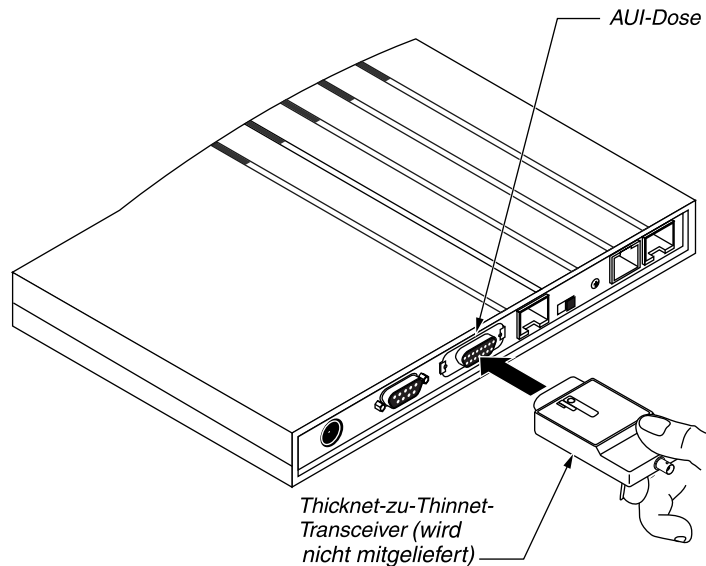
Abbildung 2-7: Anschließen des Thicknet-zu-Thinnet-Transceivers
