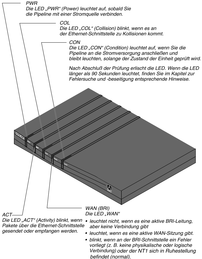
Abbildung 2-17: LEDs an der Frontblende der Pipeline
