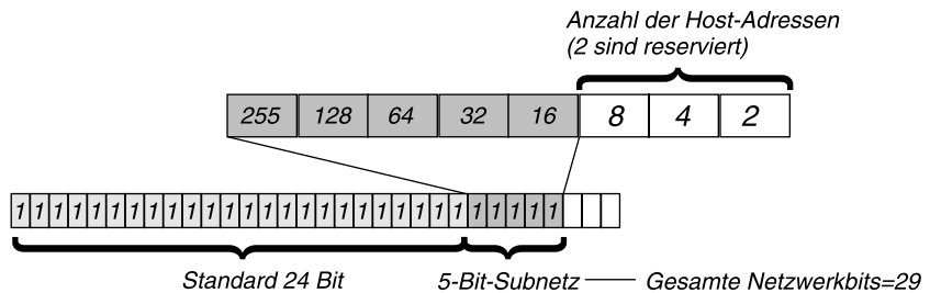
Abbildung 7-3: 29-Bit-Netzmaske und Anzahl der unterstützten Hosts
