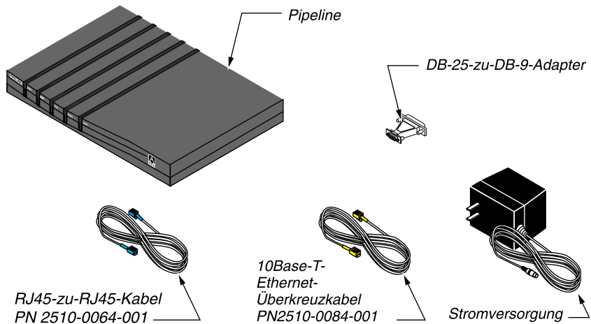
Abbildung 2-1: Hardware im Pipeline-Paket
