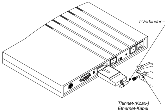
Abbildung 2-8: Anschließen des T-Verbindungsstücks und Terminators an den Transceiver
