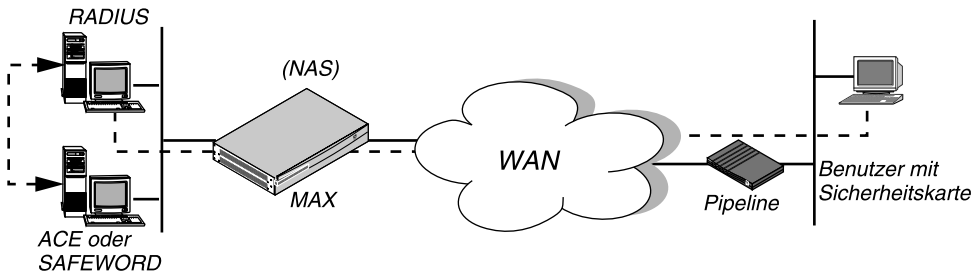
Abbildung 9-1: RADIUS-Server als Client des ACE- bzw. SAFEWORD-Servers
