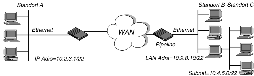
Abbildung 7-7: Verbindung über zwei Hops, die eine statische Route benötigt, wenn RIP deaktiviert wurde
