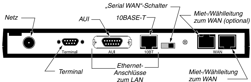
Abbildung 2-2: Rückseite der Pipeline
