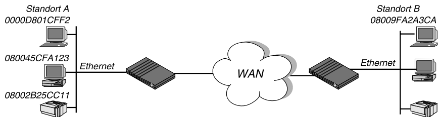
Abbildung 6-2: Erstellung einer Bridging-Tabelle durch die Pipeline
