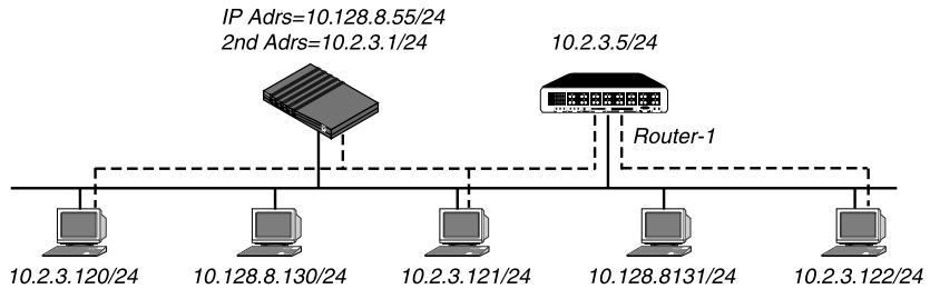
Abbildung 7-5: „Dual IP“ und gemeinsames Subnetz-Routing
