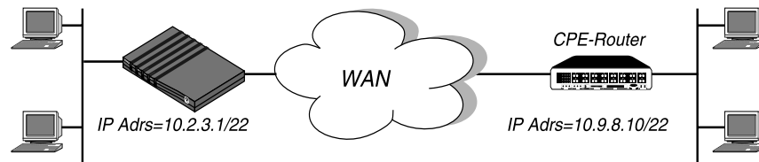
Abbildung 7-6: IP-Routing-Verbindung, die als statische Route fungiert
