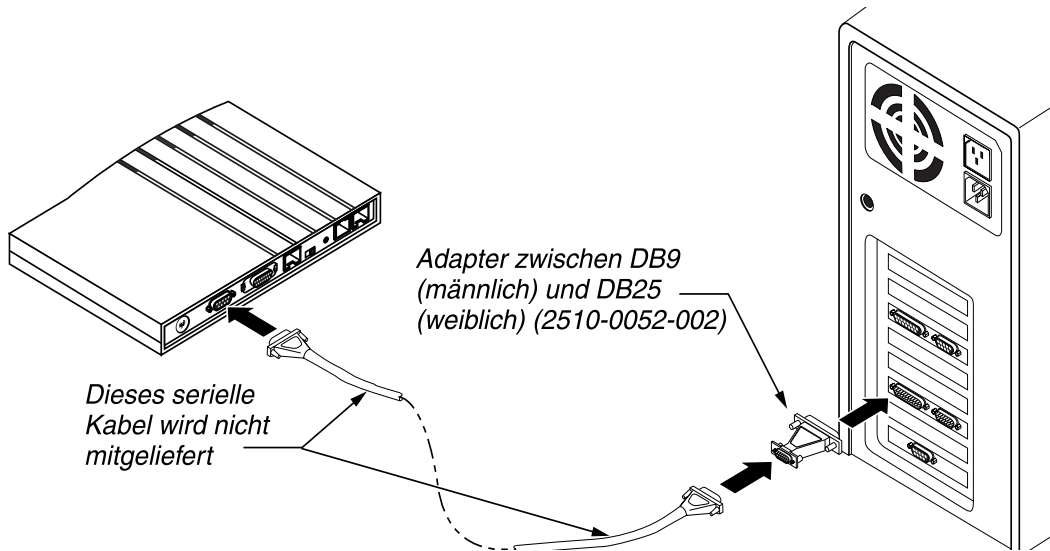
Abbildung 2-12: Anschließen des Modemkabels an den Terminal-Anschluß der Pipeline
