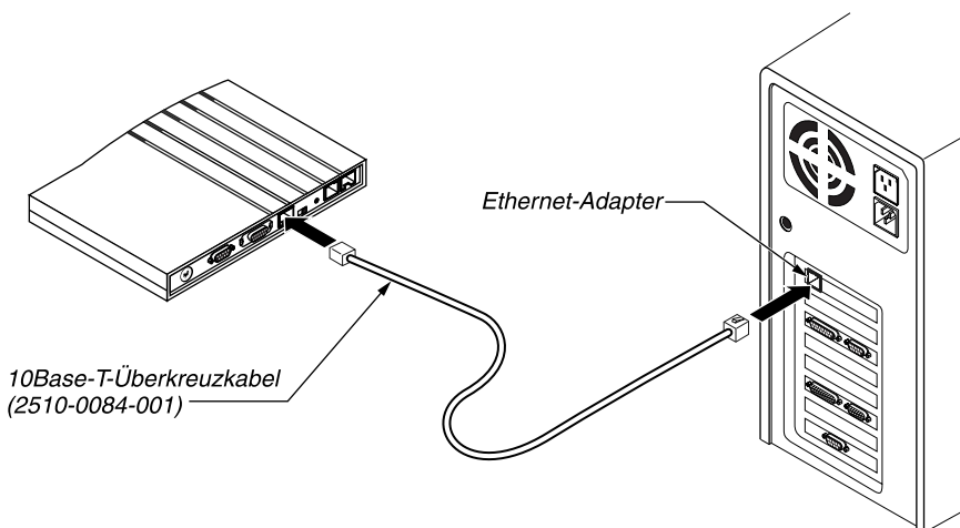
Abbildung 2-5: Anschließen der Pipeline an die Ethernet-Schnittstelle des Computers
