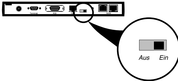
Abbildung 5-3: „On“-Position für den Schalter zur Aktivierung des seriellen WAN-Anschlusses
