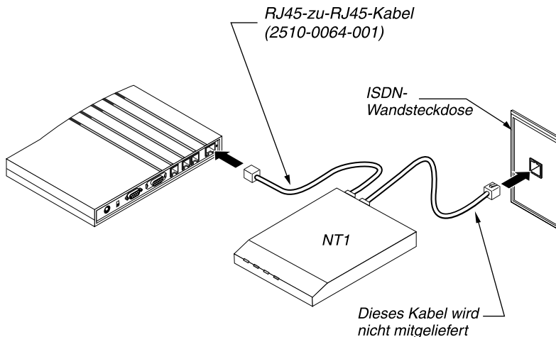
Abbildung 2-4: Anschließen einer Pipeline mit S-Schnittstelle an den ISDN-Anschluß
