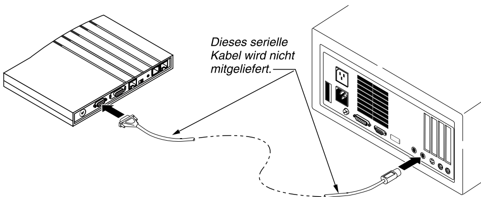
Abbildung 2-14: Anschließen eines Macintosh-Computers an den Terminal-Anschluß der Pipeline
