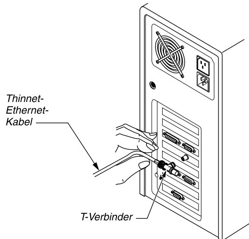
Abbildung 2-11: Anschließen des Thinnet-Kabels an das T-Verbindungsstück
